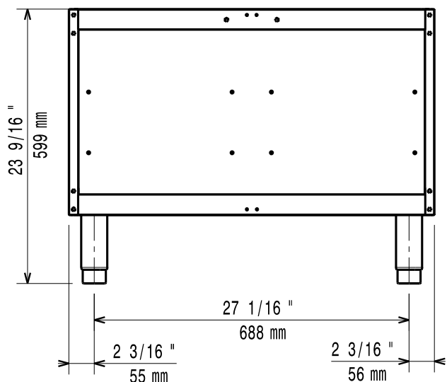
Alzado
